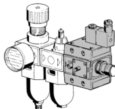
Befüllereinheit für kontrollierten Druckaufbau R1/2" Unit for controlled raise of air pressure Système d'augmentation contrôlée de la pression de l'air Sistema di aumento controllata della pressione d'aria Sistema de aumento controlado de la presión de aire
