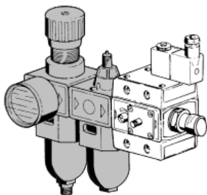
Wartungseinheit R1/2" Filter, regulator, lubricator kit Filtre, régulateur, lubrificateur Filtro, regolatore, lubrificatore Filtro, regulador, lubricador
